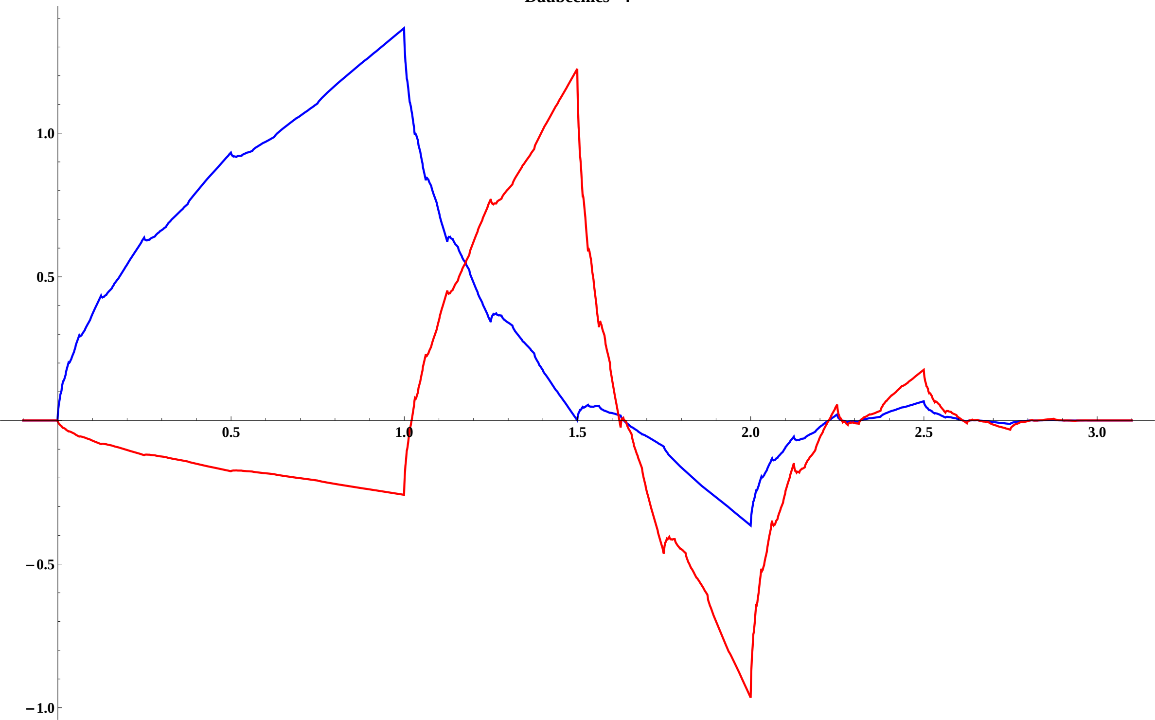
Daubechies-4
